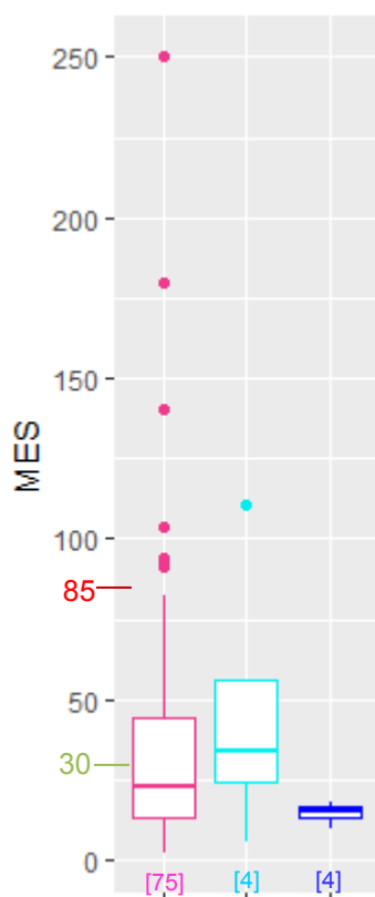
Figure 26 : Distribution des concentrations (en mg/L) du paramètre MES selon les filières de la famille CFI
