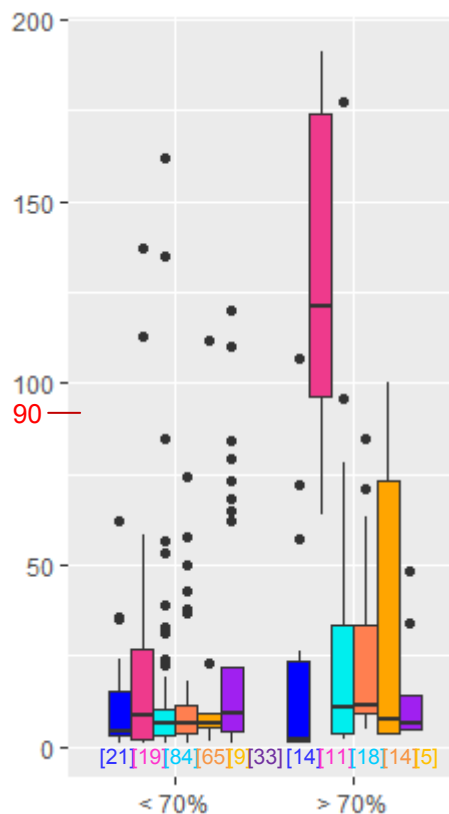
Figure 85 : Distribution des concentrations (en mg/L) du paramètre NK selon les dispositifs de la filière « lit fixe » et le taux de charge
