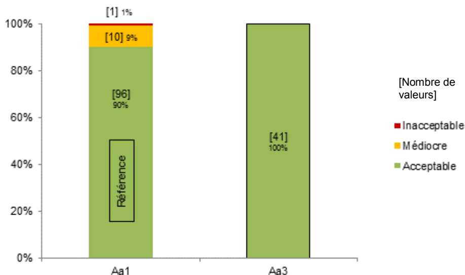
Figure 69 : Répartition dans chaque classe de qualité, selon les dispositifs de la filière « sable », des paramètres caractéristiques de l'azote
