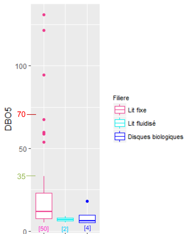
Figure 28 : Distribution des concentrations (en mg/L) du paramètre DBO 5 selon les filières de la famille CFI
