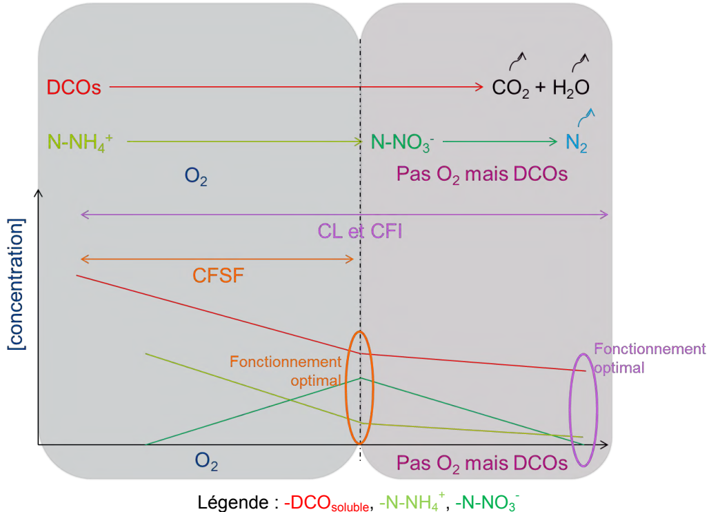
Figure 4 : Représentation schématique du traitement de la pollution dissoute
