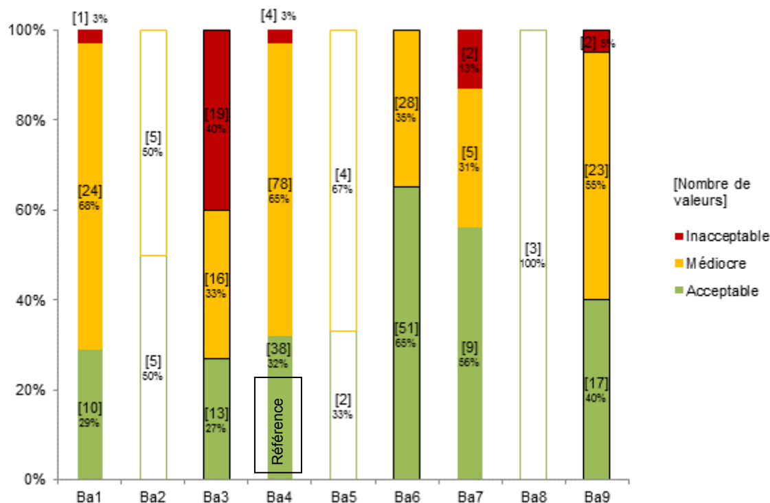
Figure 89 : Répartition dans chaque classe de qualité, selon les dispositifs de la filière « lit fixe », des paramètres caractéristiques de l'azote
